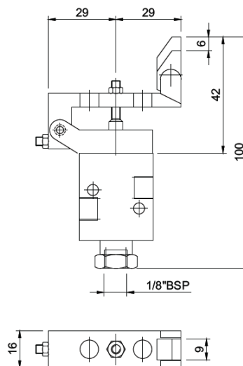
Alavanca Mola
