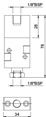
Gatilho Mola
