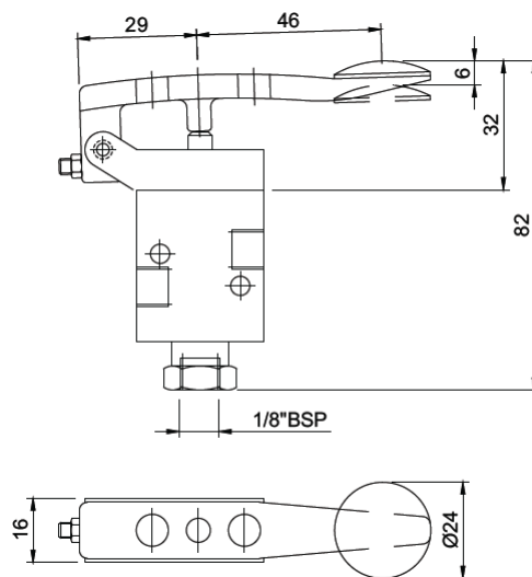
Alavanca Mola
