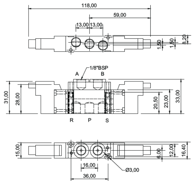
Válvula Duplo Solenoide
