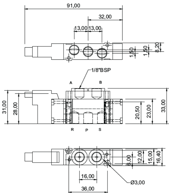
Válvula Simples Solenoide
